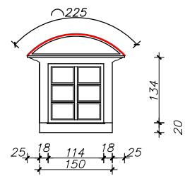
lukarna dachowa widok od strony elewacji
