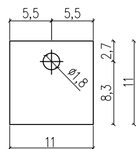
Szczegół blachy mocującej
