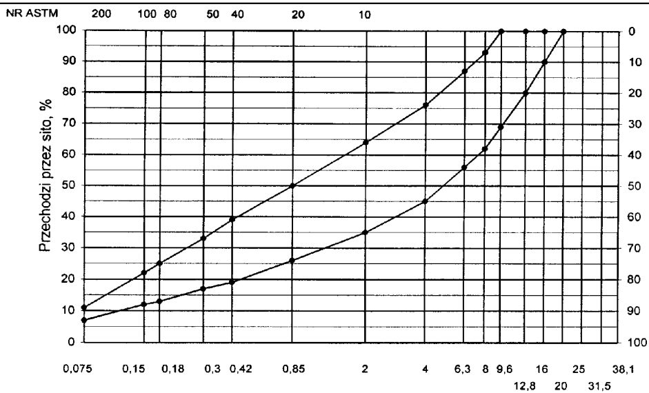
Wymiary oczek sit kwadratowych, mm graniczne uziarnienia mieszanki mineralnej BA od 0 do 16mm, od 0 do 12,8 mm do warstwy ścieralnej nawierzchni drogi o obciążeniu ruchem KR1 lub KR2
