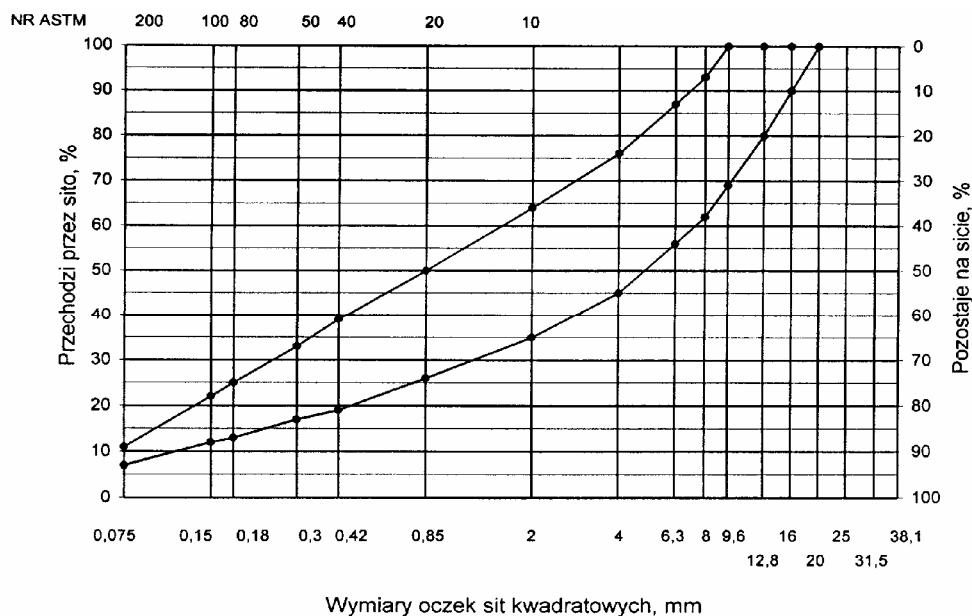
Rys. 1. Krzywe graniczne uziarnienia mieszanki mineralnej BA od 0 do 16mm, od 0 do 12,8 mm do warstwy ścieralnej nawierzchni i drogi o obciążeniu ruchem KR1 lub
