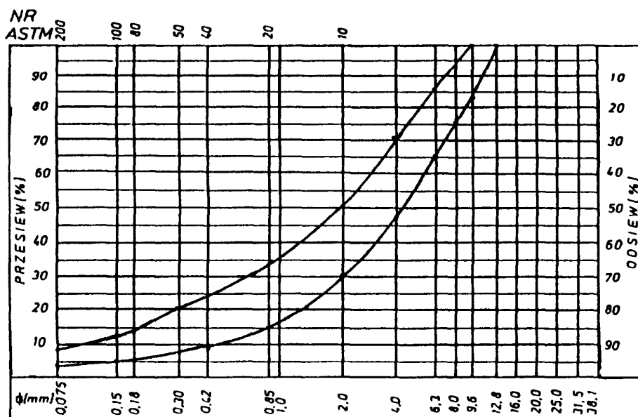
graniczne uziarnienia mieszanki mineralnej 0,12,8 mm do podbudowy z betonu asfaltowego dla KR 1-2
