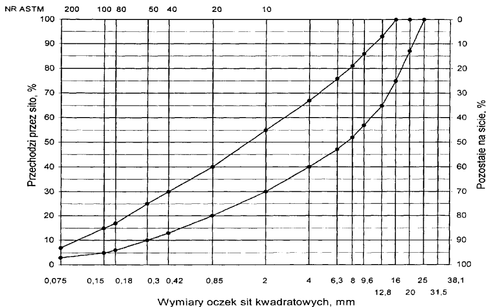
Rys. 2. Krzywe graniczne uziarnienia mieszanki mineralnej BA od 0 do 20 mm do warstwy wiążącej
