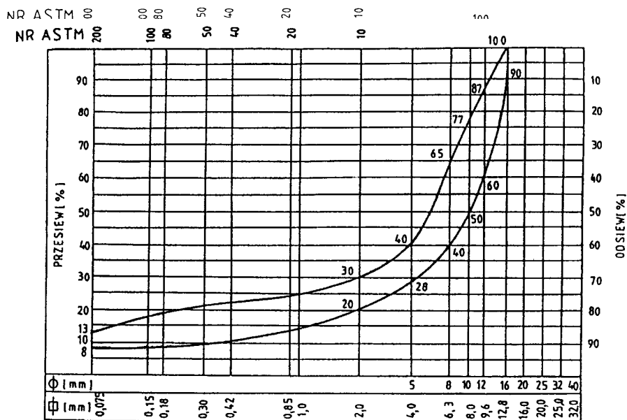
Rys. 5. Krzywe graniczne uziarnienia mieszank mineralnych SMA od 0 mm do 12,8 mm
