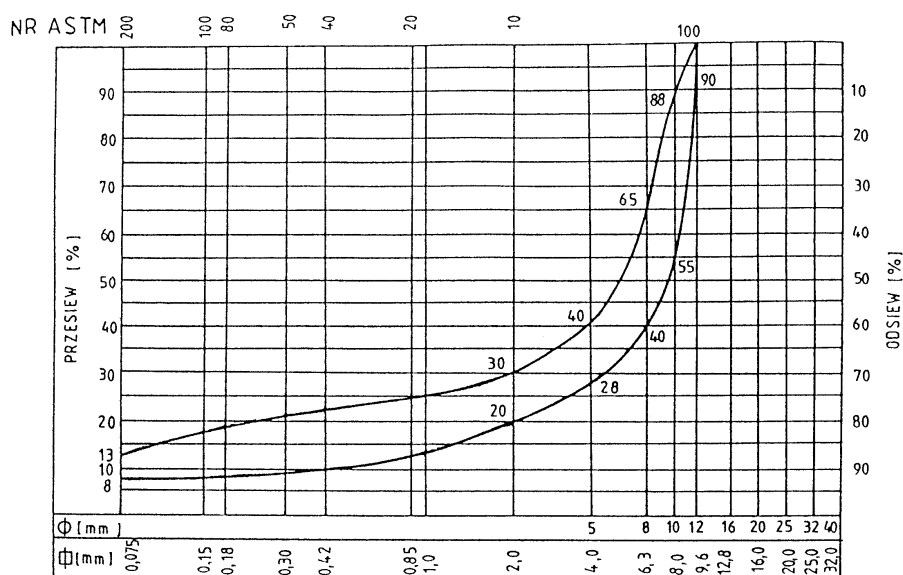
Rys. 3. Krzywe graniczne uziarnienia mieszanek mineralnych BA od 0 mm do 8
