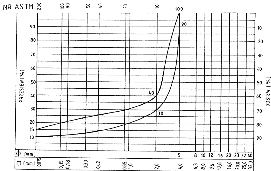
Rys. 3. Krzywe graniczne uziarnienia mieszanek mineralnych BA od 0 mm do 8 mm
