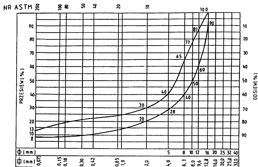
Rys. 5. Krzywe graniczne uziarnienia mieszank mineralnych BA od 0 mm do 12,8 mm
